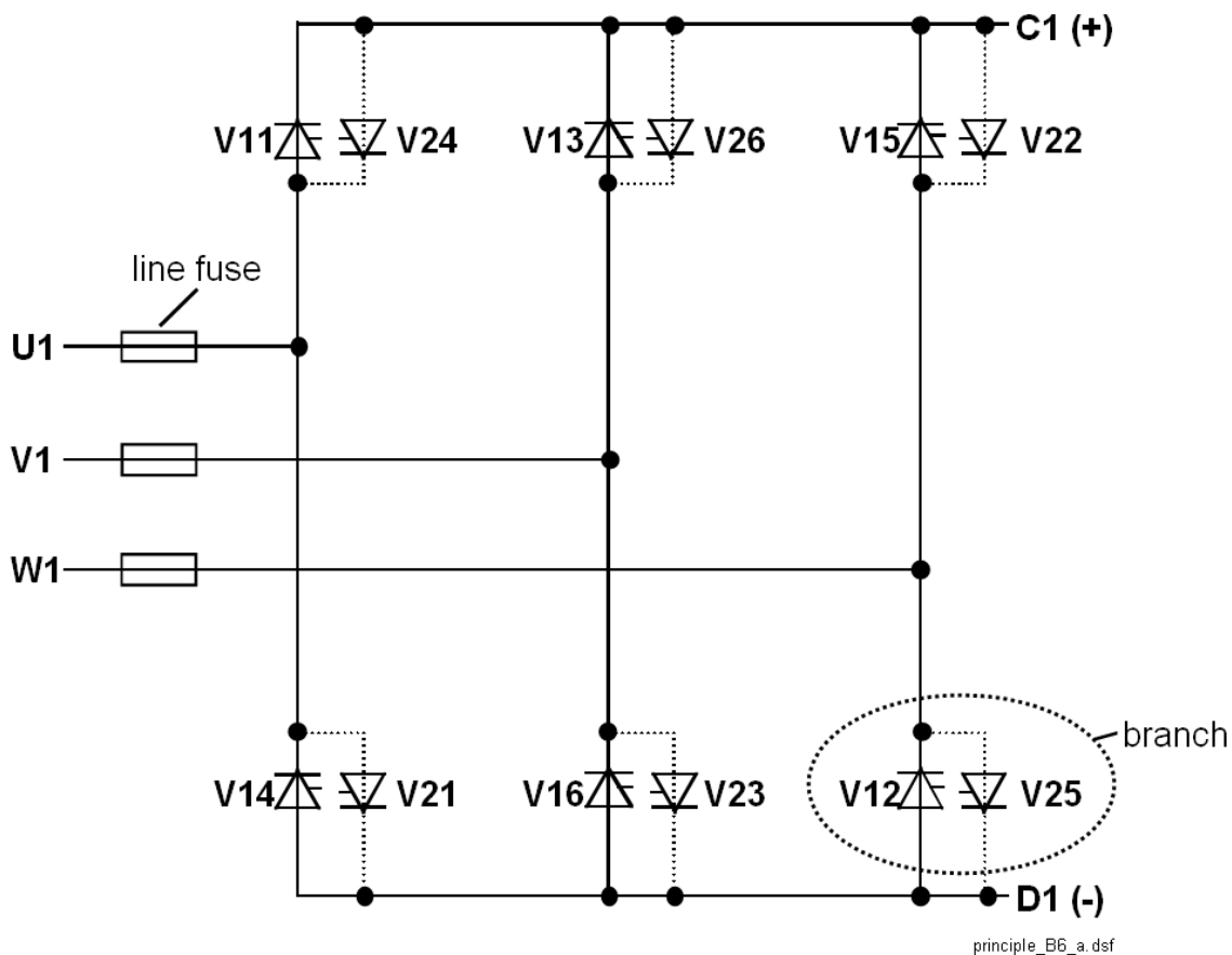
Bridge configuration D1 to D4
