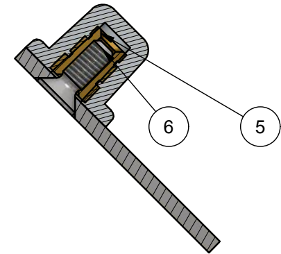
B-B (2 : 1)
