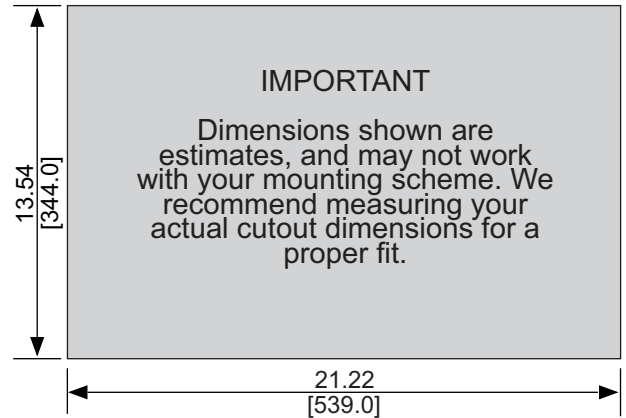
Cutout Dimensions
