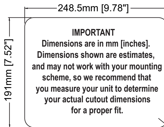
Cutout Dimensions
