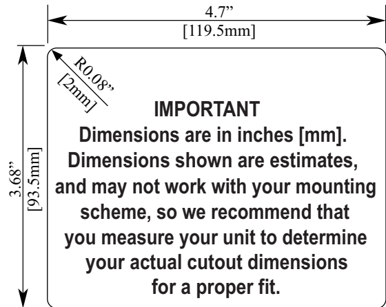
Cutout Dimensions
