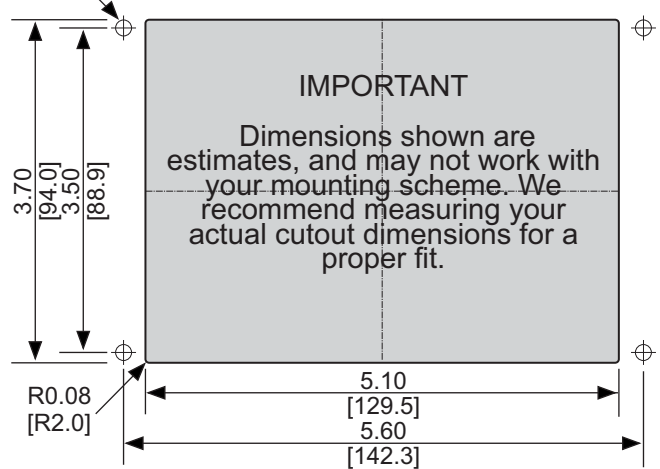
Cutout Dimensions
