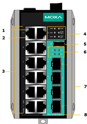
EDS-G516E-4GSFP
