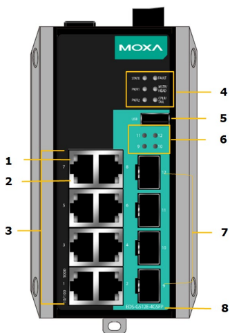
EDS-G512E-4GSFP
