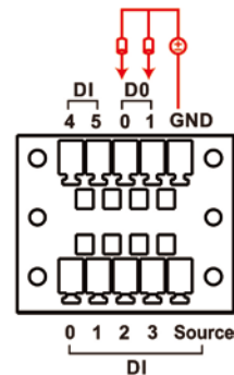
DO Wiring
