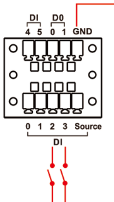
DI Dry Contact Wiring
