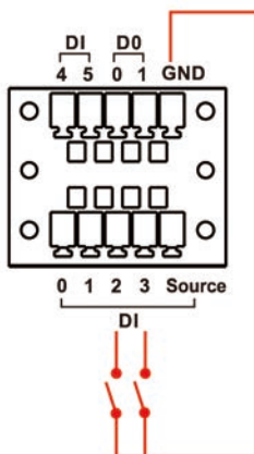
DI Dry Contact Wiring
