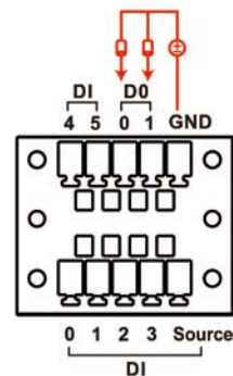
DO Wiring
