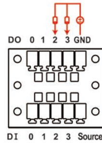
DO Wiring
