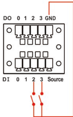
DI Dry Contact Wiring
