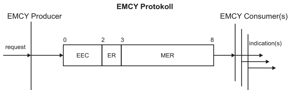
Fig. 5-10:EMCY Protocol
