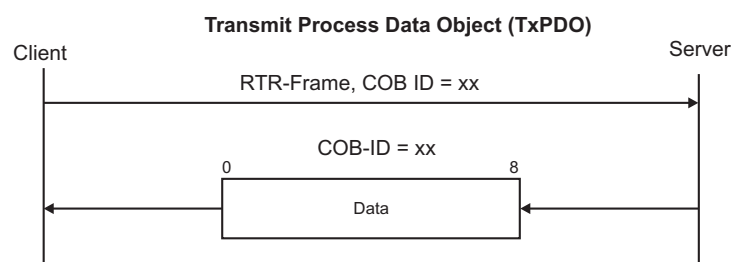
Fig. 5-2:TxPDO
