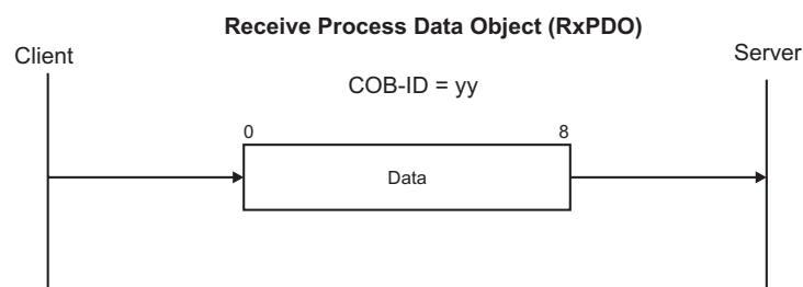
Fig. 5-1:RxPDO
