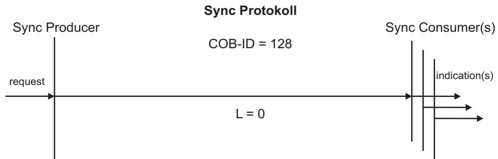
Fig. 5-9:SYNC Protocol
