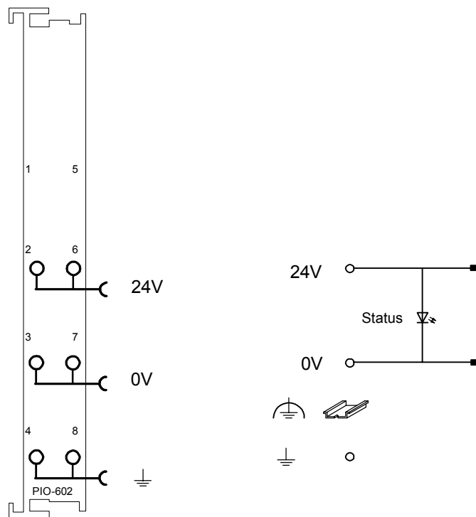
Fig. 4.12.4-1: Supply Module PIO-602
