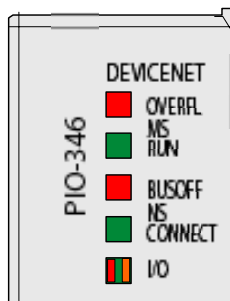
Fig. 3-4: Display elements
