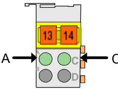
Fig. 4.9.3-1: Display Elements
