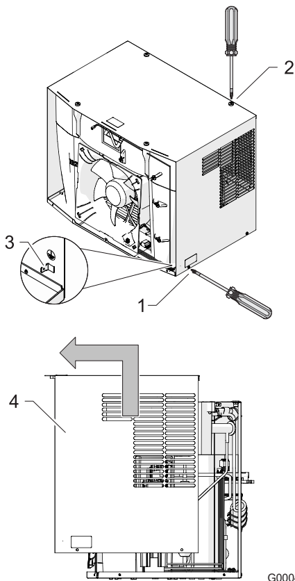
Abb. 18: Gerätehaube entfernen
