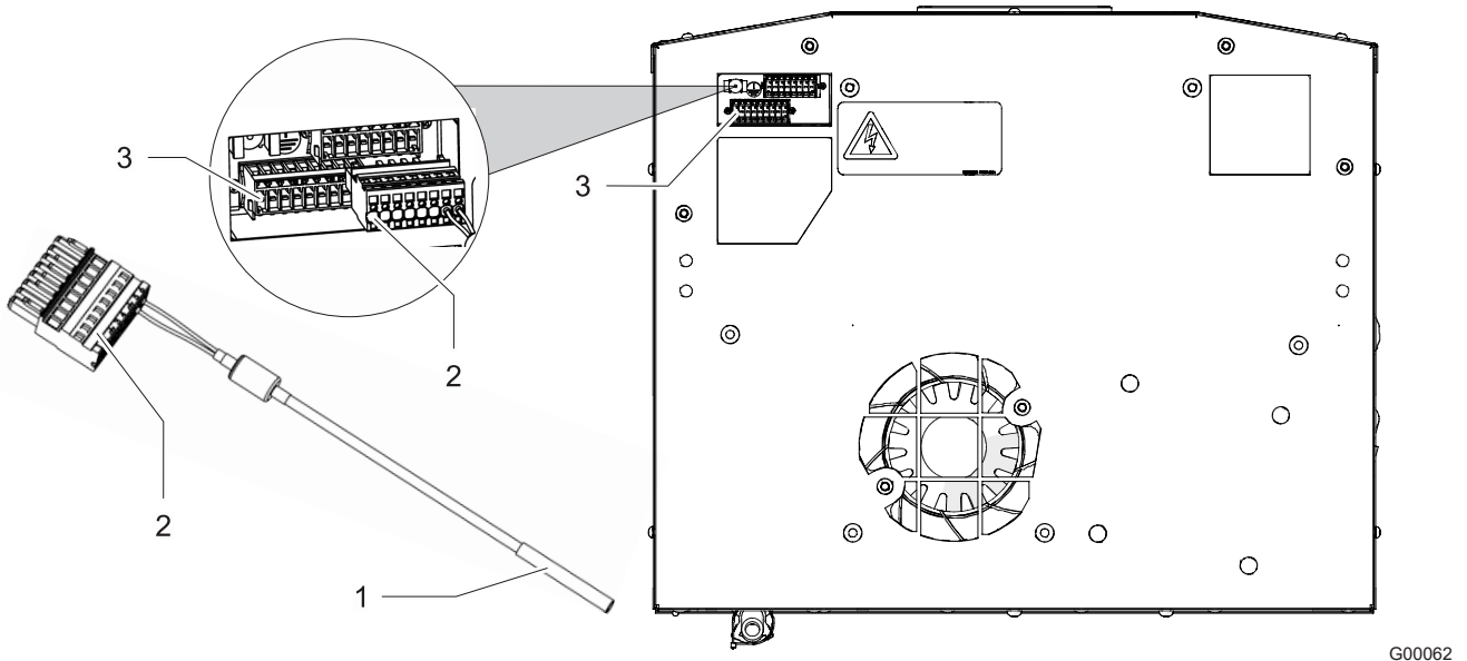
Fig. 23: Sonda di temperatura - TS2
