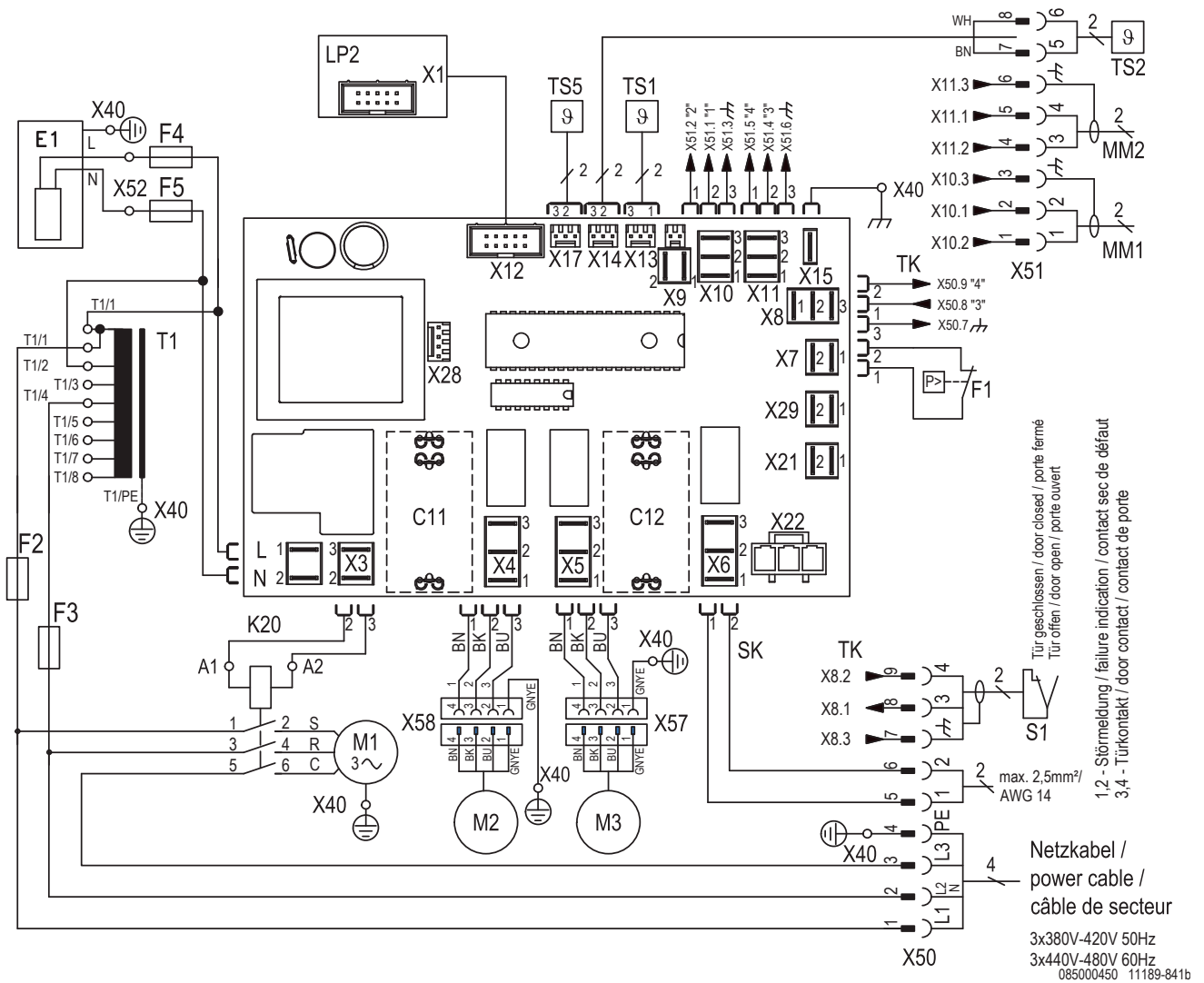
Abb. 21: Stromlaufplan
