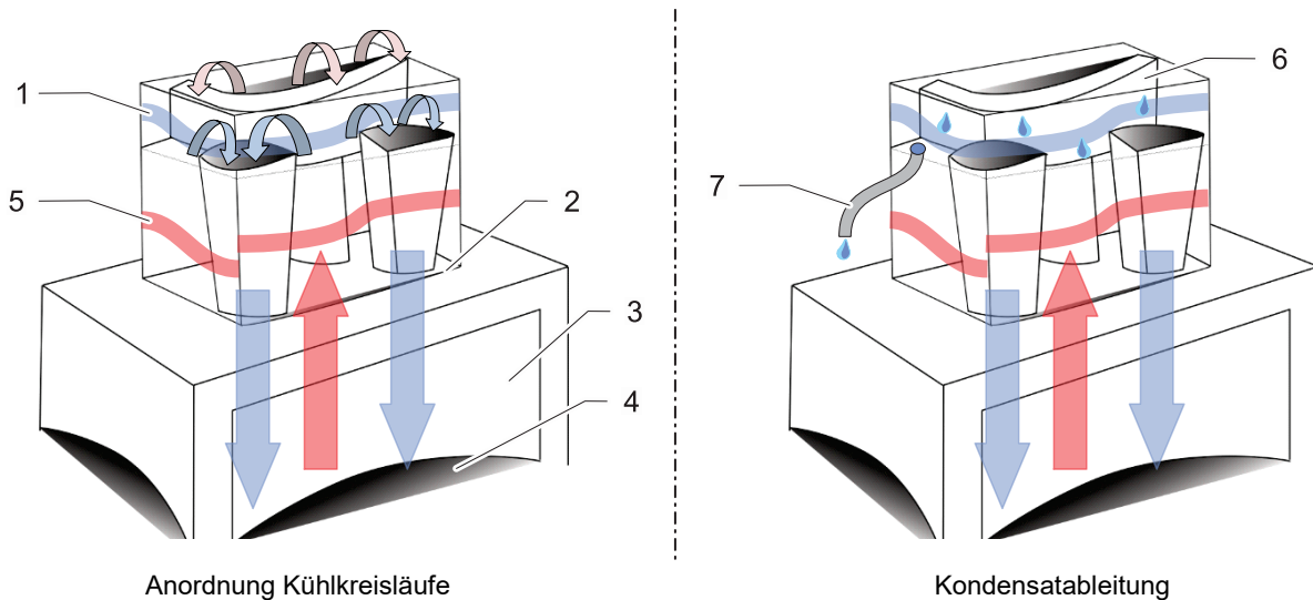
Abb. 8: Kühlkreisläufe und Kondensatableitung
