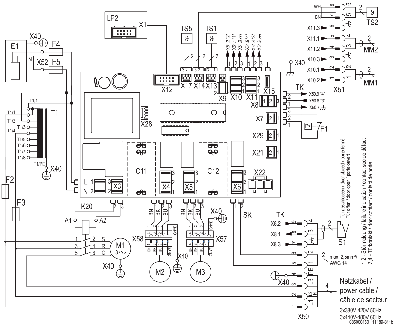
Fig. 21: Esquema eléctrico
