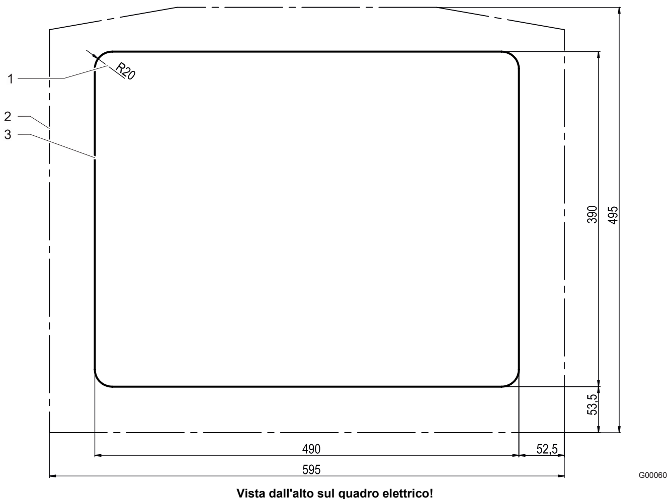
Fig. 14: Apertura nel quadro elettrico
