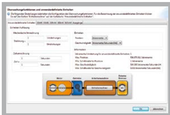
Configuration of PSSu K F EI
