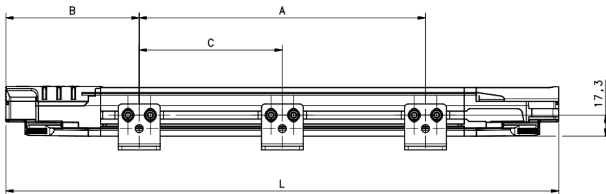
Fig. 19 – Light curtain dimensions
