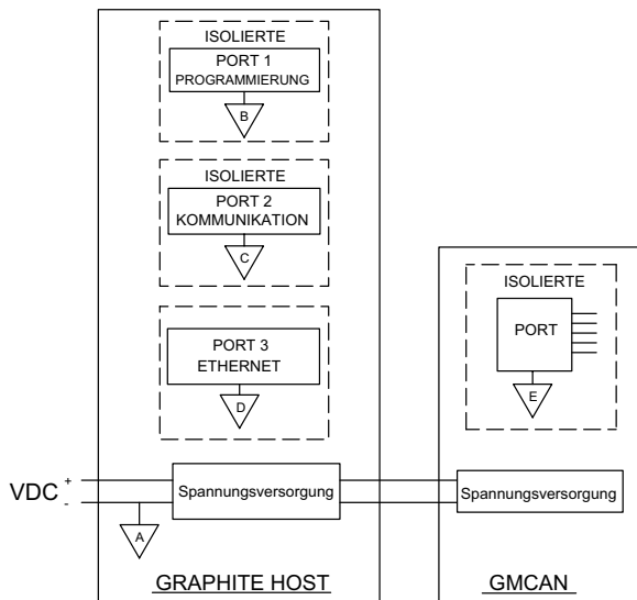
Blockschaltbild zur GMCAN
