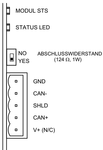
Abbildung 3. GMCAN PINBELEGUNG DER SCHNITTSTELLE
