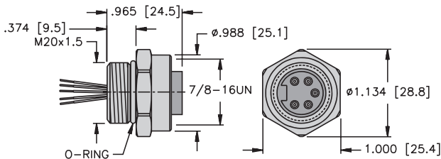
P-RKF .. M20
