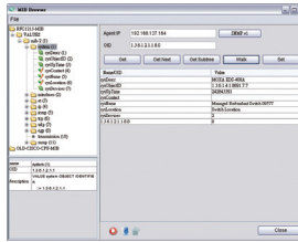
MIB Browser
